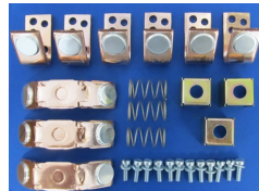
Contactos Lovato
